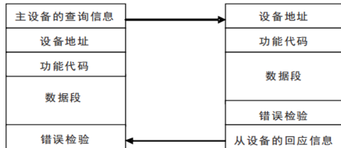
图 3 Modbus 通讯方式
