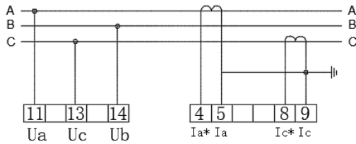
三相三线电流互感器直接接入
