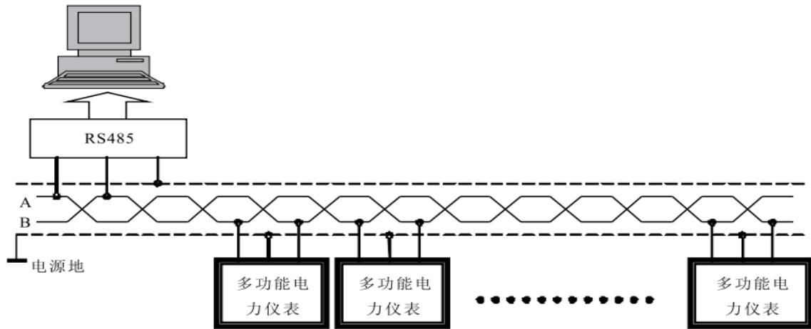
图2 T型网络的连接方式
