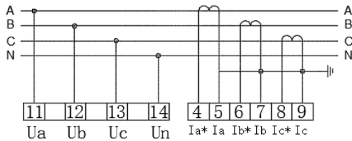
三相四线电流互感器接入
